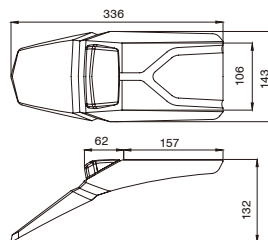
ANATO ED REAR FENDER KIT
